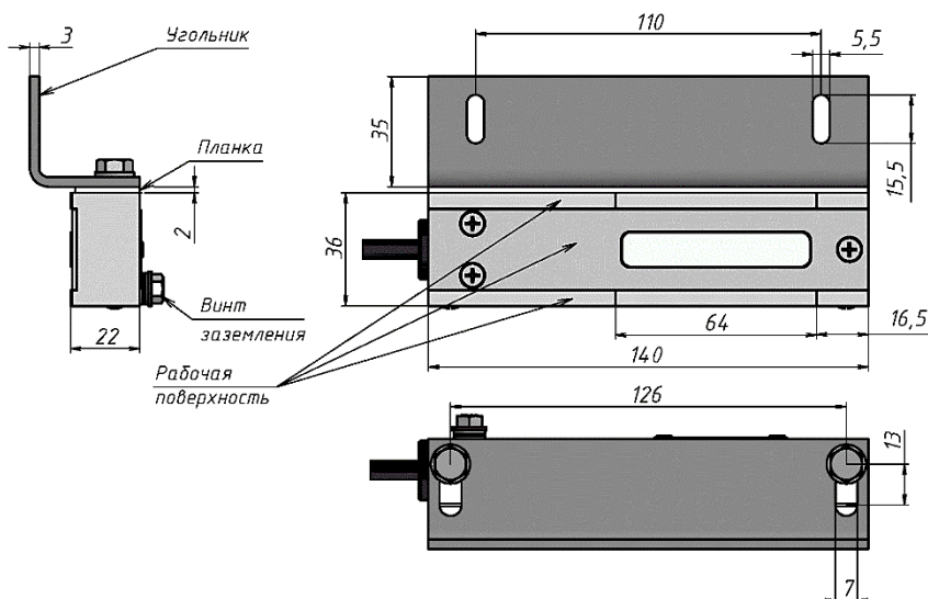
Рисунок 4 - Корпусная часть
