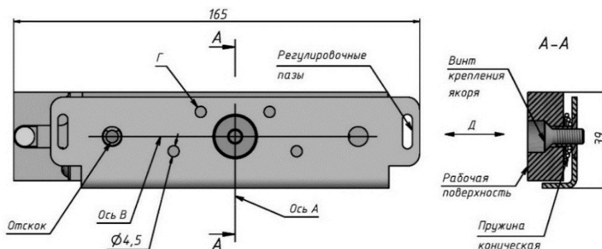
Рисунок 10 - Якорная часть замка варианта «G»
