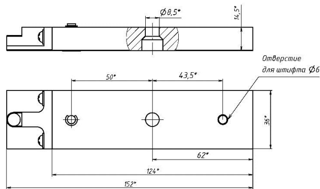
Рисунок 7- Габаритный чертеж якоря
