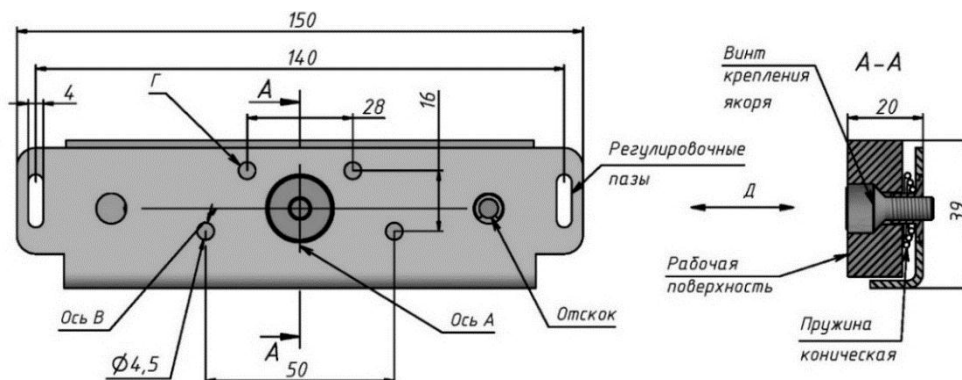
Рисунок 9- Якорная часть замка варианта «Н»
