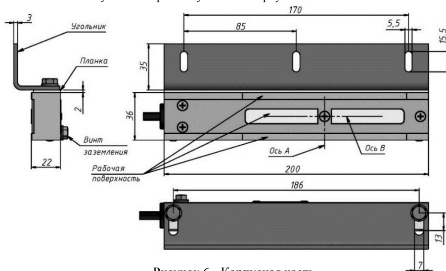
Рисунок 6 - Корпусная часть
