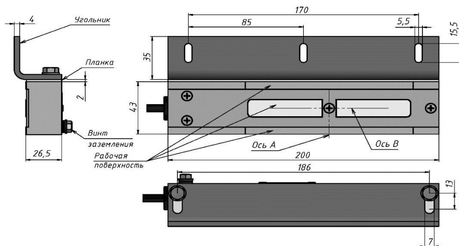
Рисунок 4 - Корпусная часть
