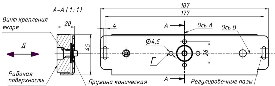
Рисунок 5 - Якорная часть замка варианта «Н»
