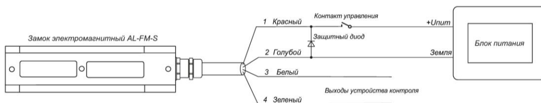
Рисунок 7- Схема подключения замка
