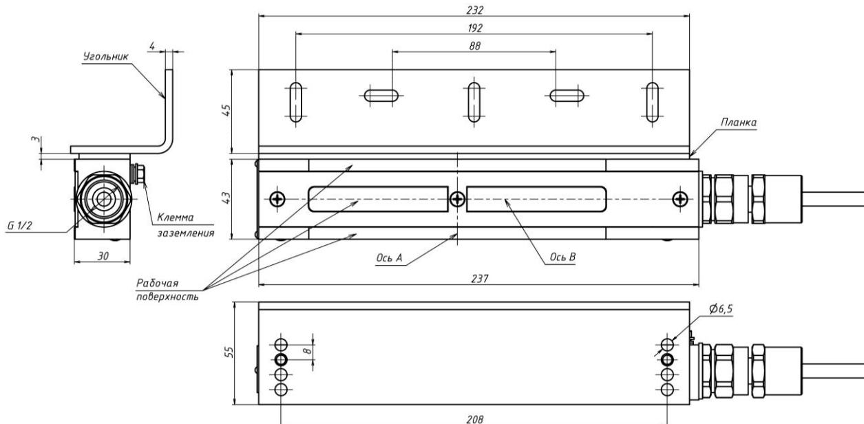
Рисунок 4 - Корпусная часть
