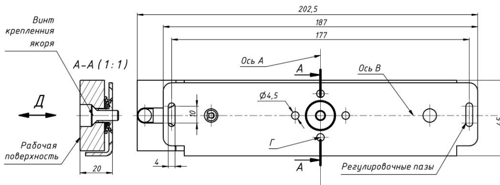
Рисунок 6 - Якорная часть замка варианта «Г»
