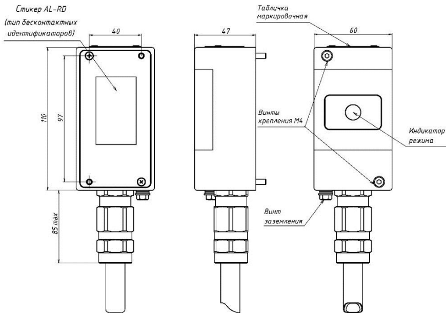
Рисунок 1 - Габаритно-установочные размеры счетчика AL-RD-S04-NRU
