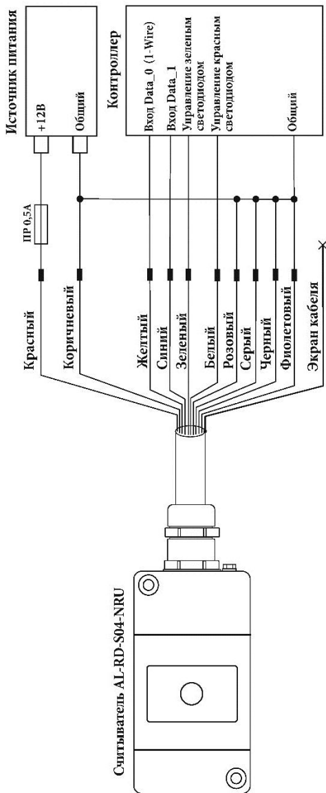
Рисунок 2 - Схема подключения считывателей AL-RD-S04-NRU-К, AL-RD-S04-NRU-М и AL-RD-S04-NRU-Т к контроллеру СКУД. При установке интерфейса 1-Wire (Эмуляция «touch memory») вывод кабеля «синий» остается свободным.
